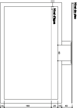
TANQUE DE CONTATO CORTE - ESC. 1:25
