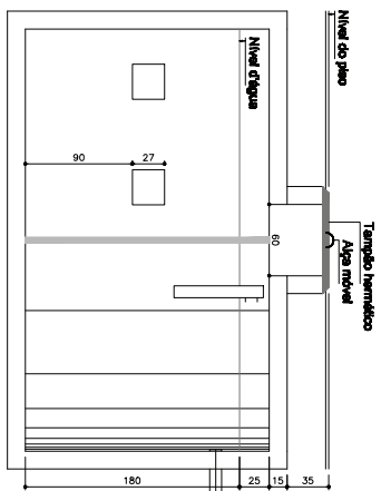
FILTRO AERADORIO CORTE - ESC. 1:25
